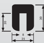
Typ G Kantenschutz
