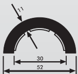
Typ F30 Rohrschutz
