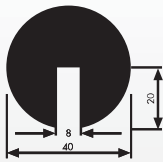
Typ B Kantenschutz
