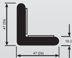
Typ H (Typ H1,9) Eckschutz
